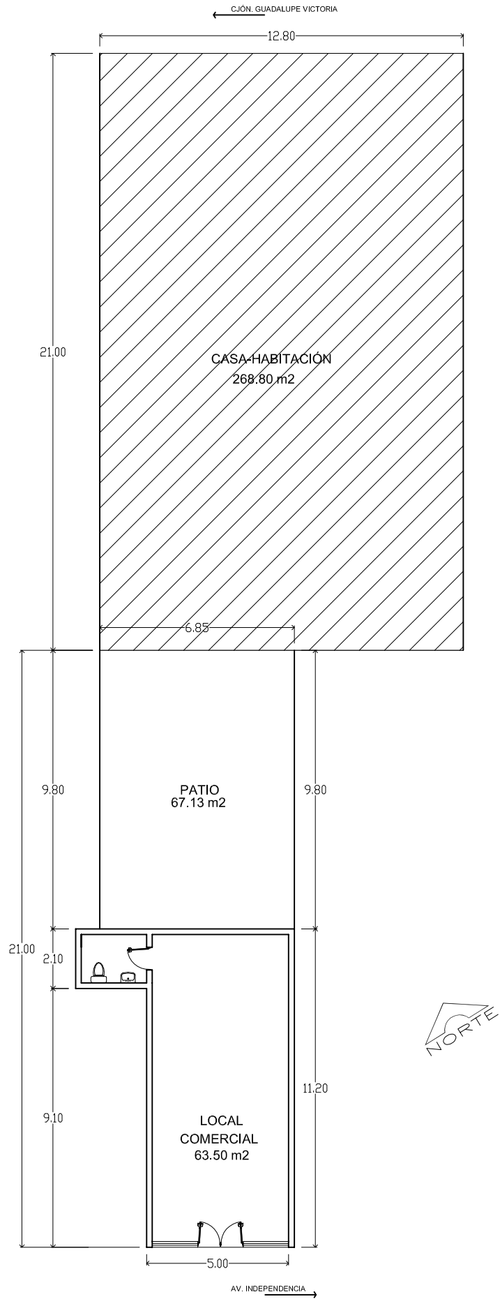
PLANTA ARQUITECTÓNICA
