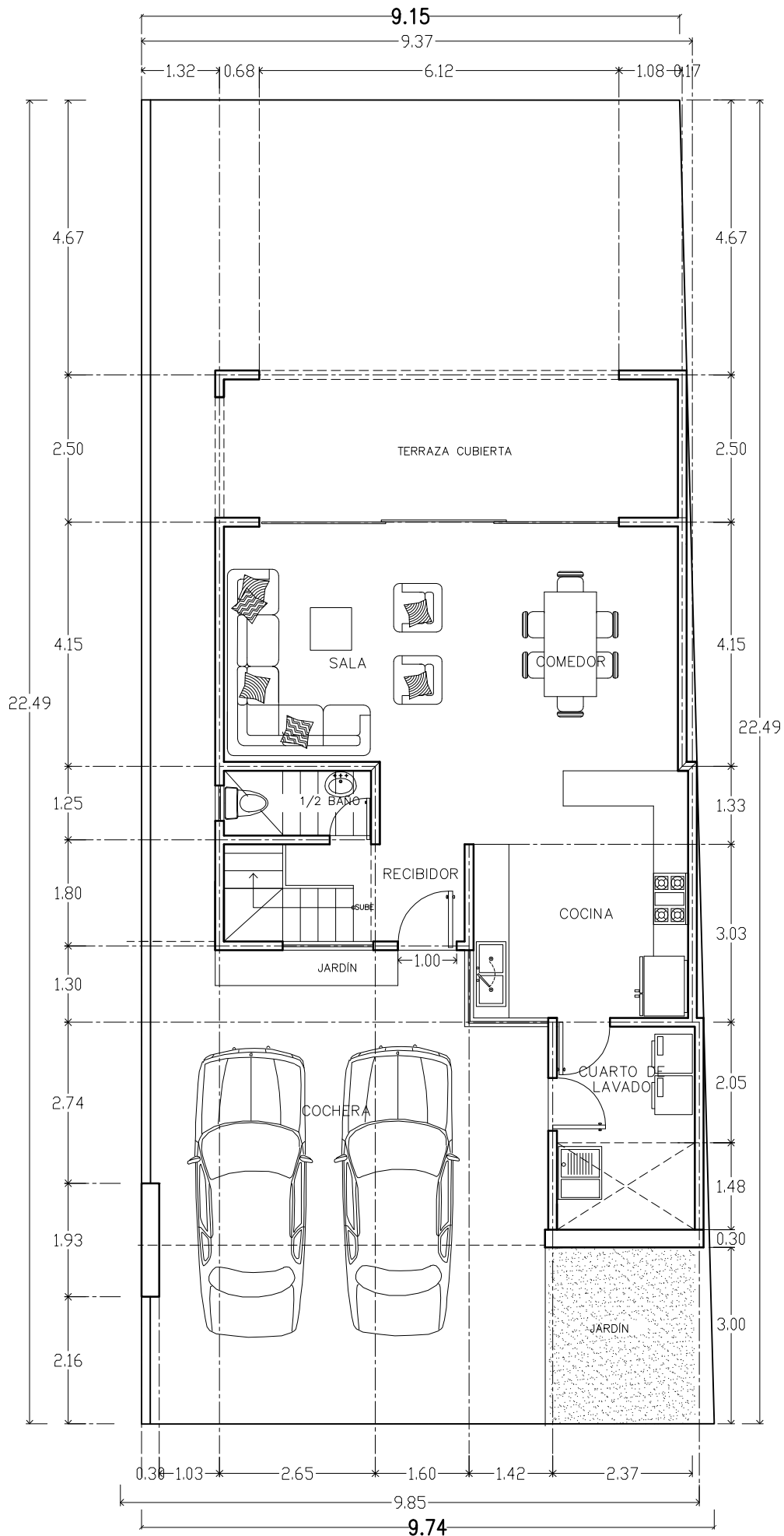
PLANTA ARQUITECTÓNICA BA 1A 127.87 M2
