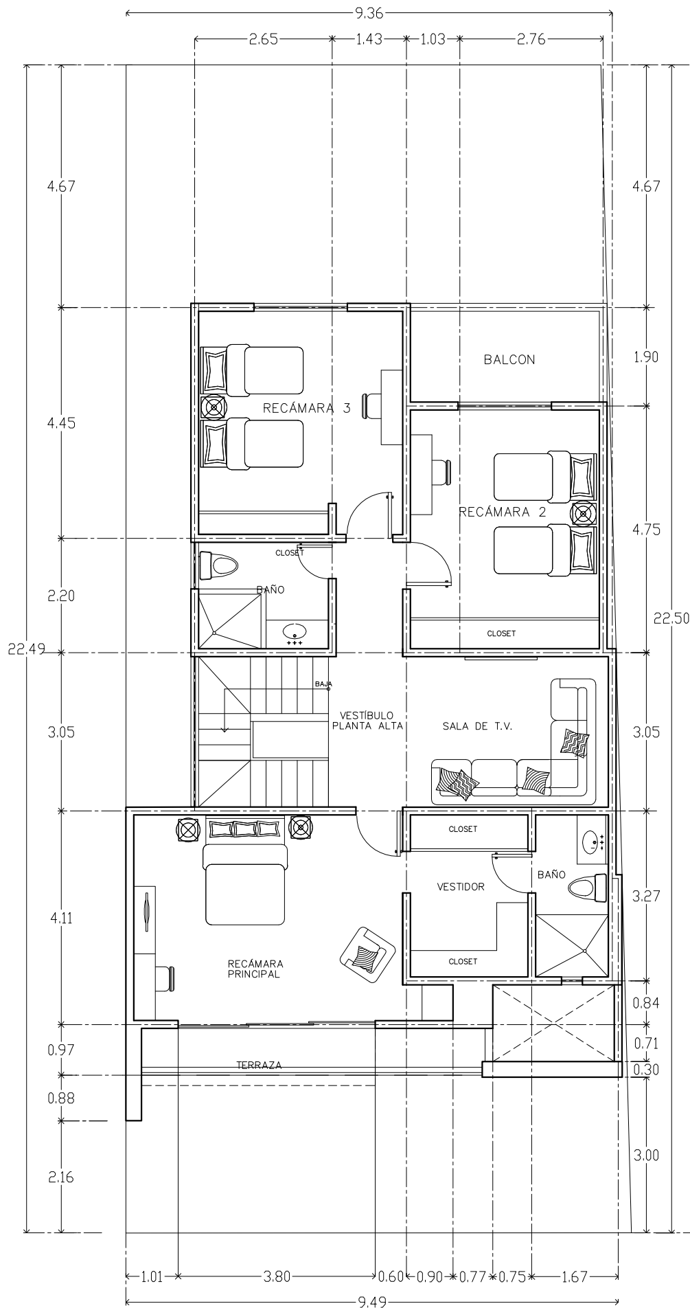
PLANTA ARQUITECTÓNICA ALTA 115.10 M2
